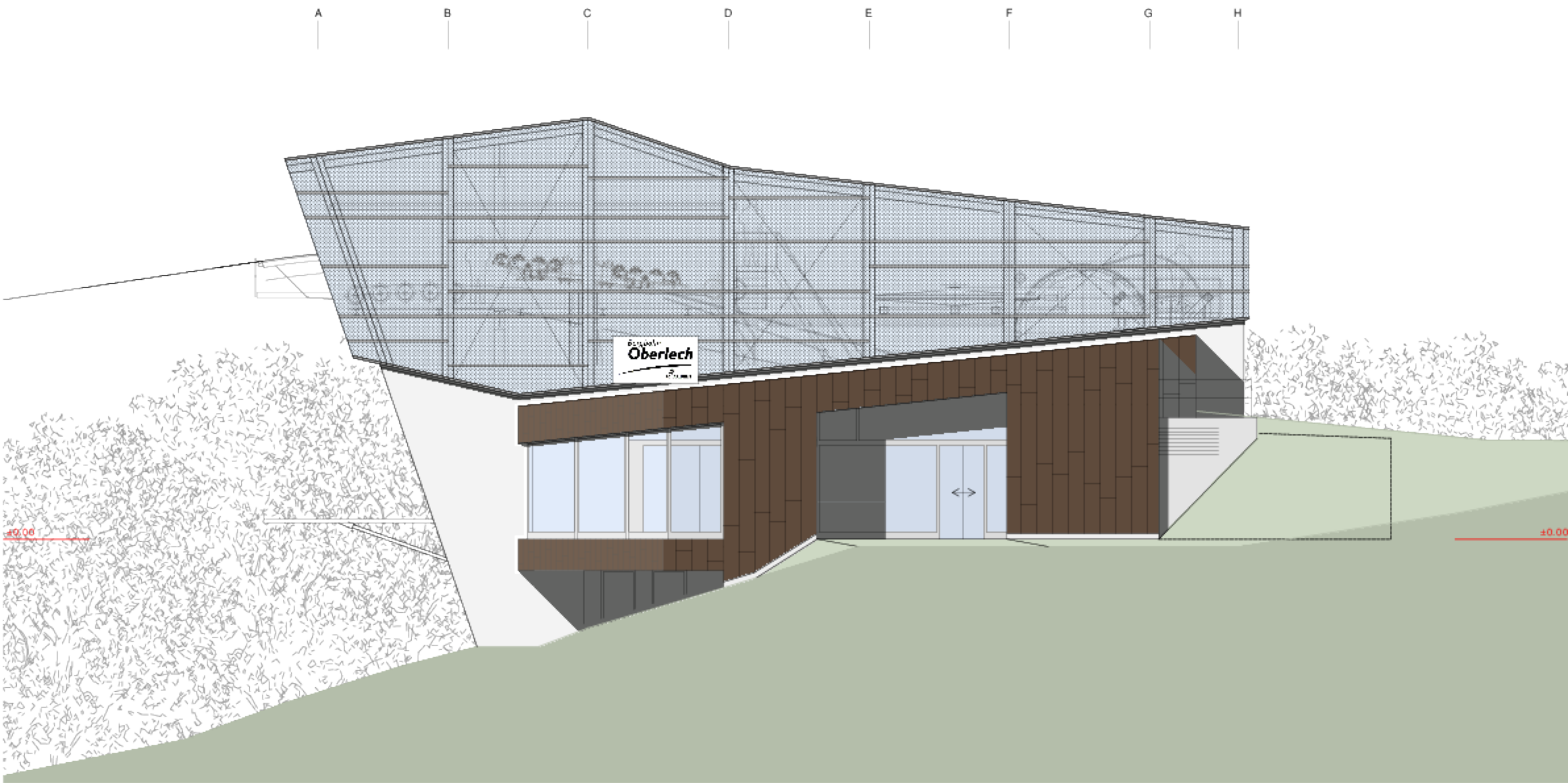
ANSICHT VON NORDOSTEN
